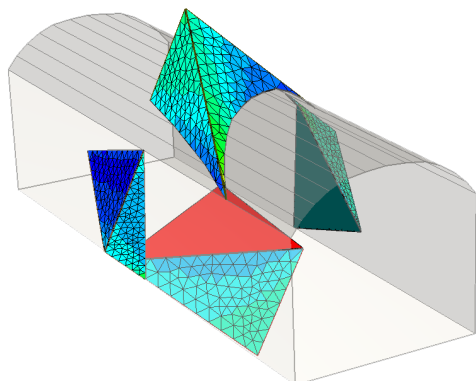
3D 模型场应力等值线视图
