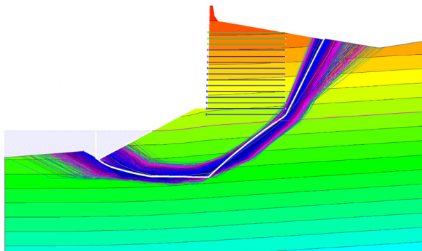
Slide2边坡稳定性和渗流分析结果
