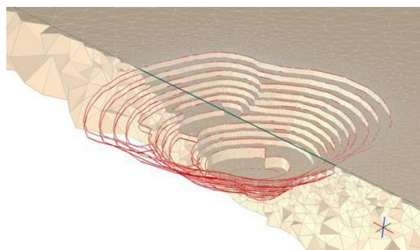
露天矿的开采平面
