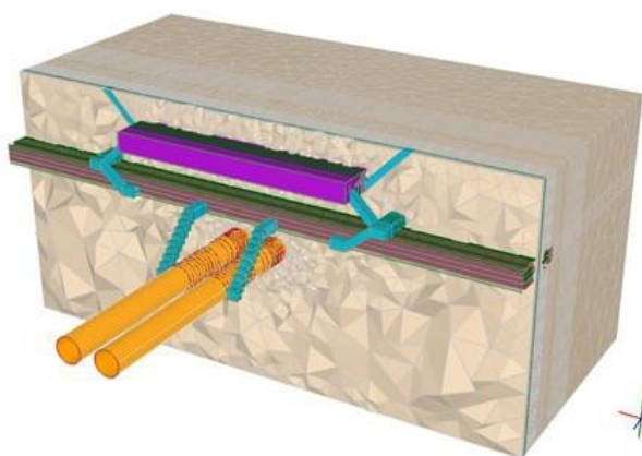
地铁隧道施工模型
