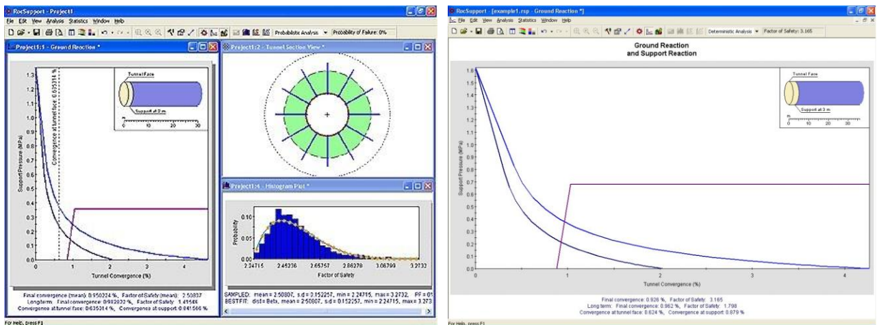
地表效应曲线（短期和长期）和支护效应。这些曲线的交点决定了支护的安全系数
