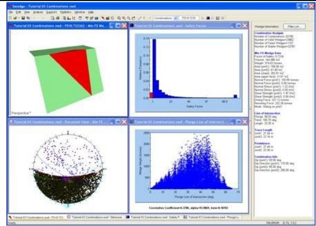
岩质边坡楔体稳定失效概率分析：直方图、散点图、立体网络图；加固和楔形体组合分析
