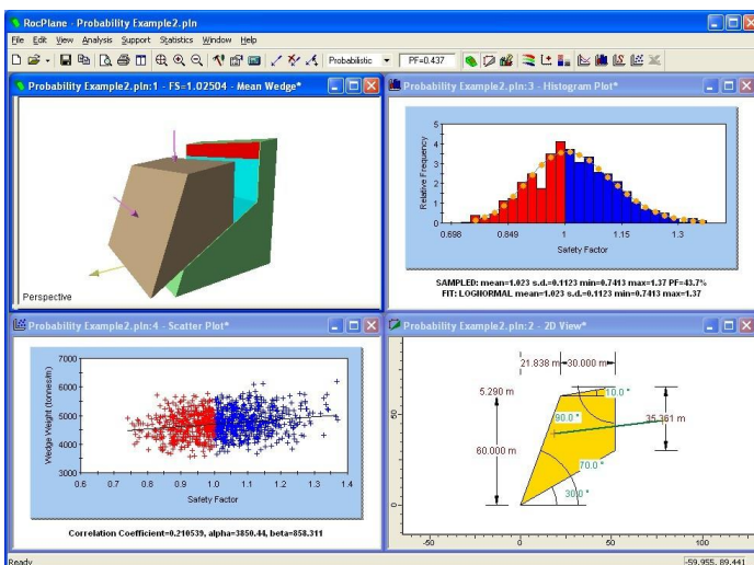
概率分析结果可以绘制成直方图显示或散点图，破坏楔形体的数据以红色高亮显示
