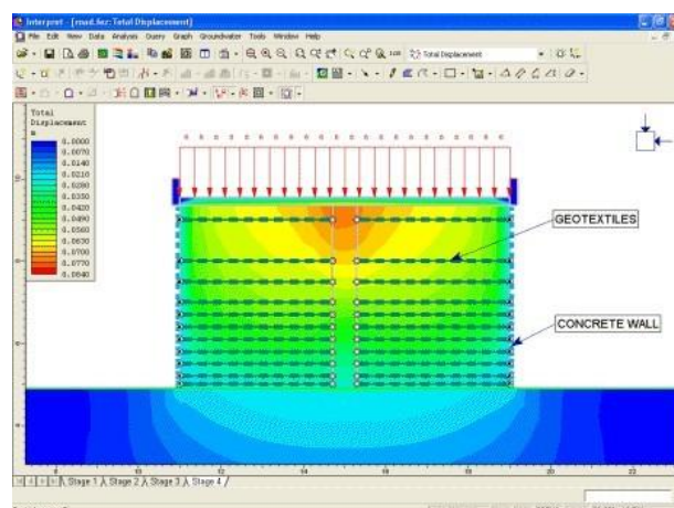
土工合成材料加筋土
