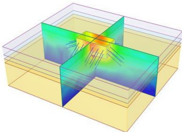
三维支护开挖
