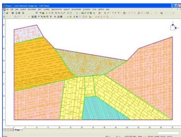
RS 2 可以用于分析露天矿坑，模拟分步开挖，能够批量定义各种类型的交叉节理构造
