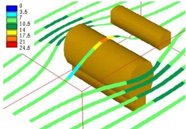
主应力等值面、围绕两个地下洞室的主应力迹线
