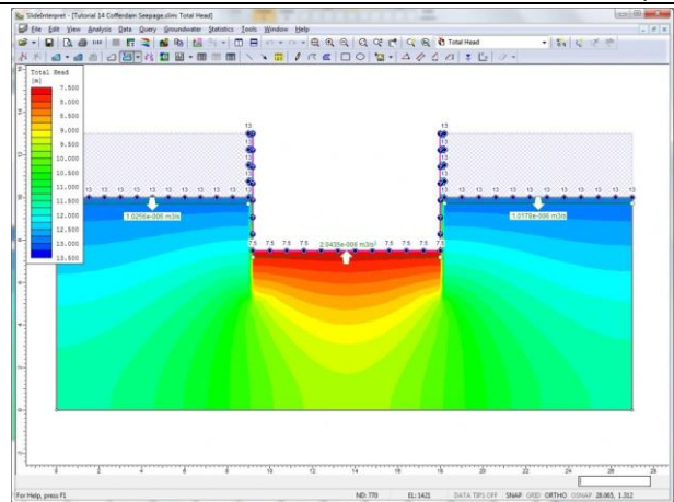
围堰渗流分析
