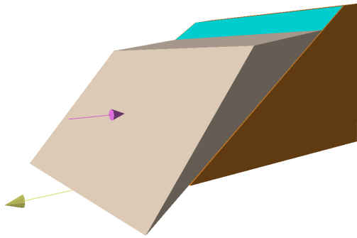
受水压力和地震力作用下沿张拉裂缝滑动的岩质边坡平面
