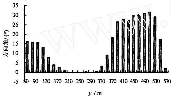
图2 主滑方向统计图
