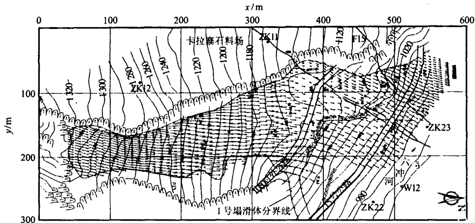
图1 塌滑体滑动方向
