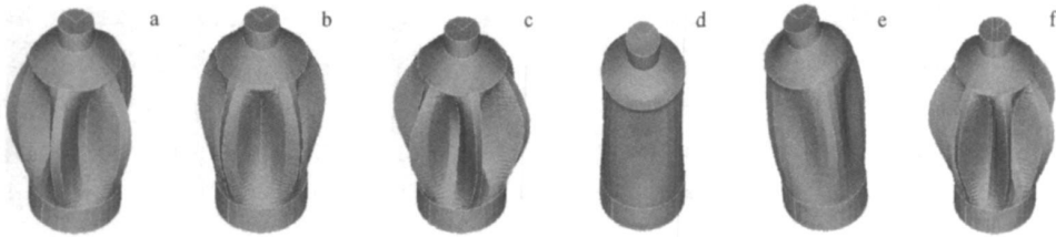
图3 容器不同模式下的振形图
