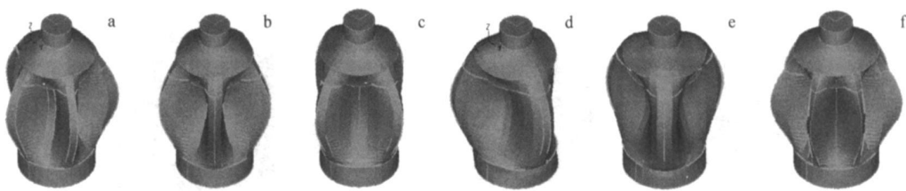
图 5 耦合振动下的不同模式振形图
