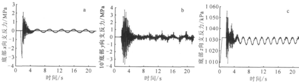
图 10 容器底部支撑处不同方向的支反力 Fig. 10 Support reaction at different direction of bottom of vessel a—x 方向; b—y 方向; c—z 方向
