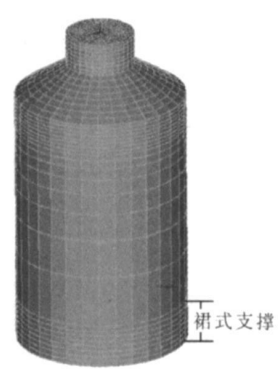
图 1 快堆主容器 ADINA 模型 Fig. 1 ADINA model for main vessel of FBR
