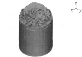
图4 液体晃动的 1 阶模态振形图
