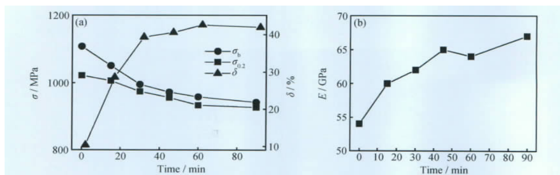
图 7 冷轧态合金在 650℃ 下退火不同时间后的力学性能 (a)强度和伸长率;(b)弹性模量
