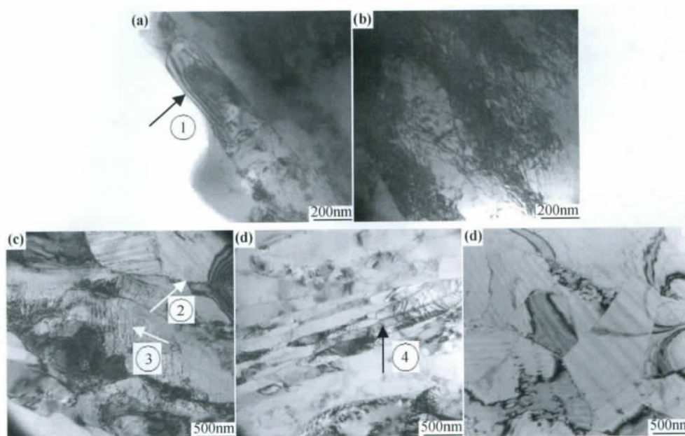
图 5 冷轧态合金在 650^\circ\text{C} 下退火不同时间后的 TEM 组织 (a)和(b)15min; (c)和(d)45min; (e)90min
