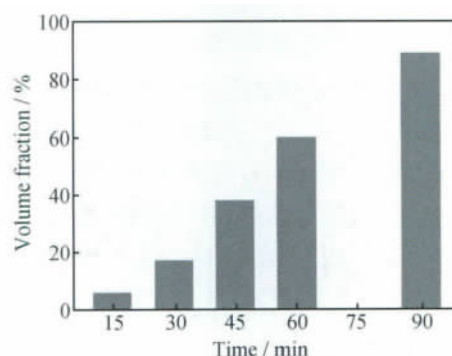
图 4 退火时间对再结晶体积分数的影响
