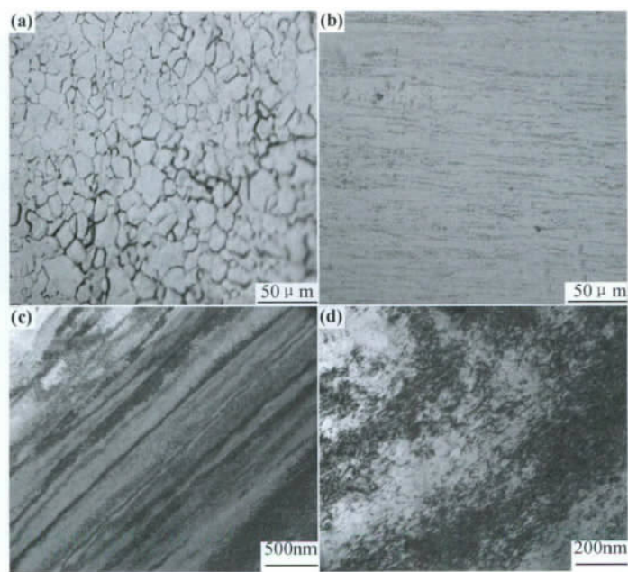
图 1 固溶态和冷轧态 Ti-35Nb-9Zr-6Mo-4Sn 的显微组织
