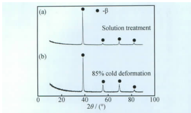
图 2 固溶态(a)和 85%(b)形变冷轧态合金的 XRD 图谱
