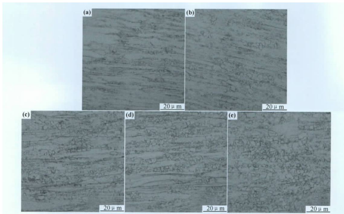
图 3 冷轧态合金在 650℃ 退火不同时间的光学显微镜照片
