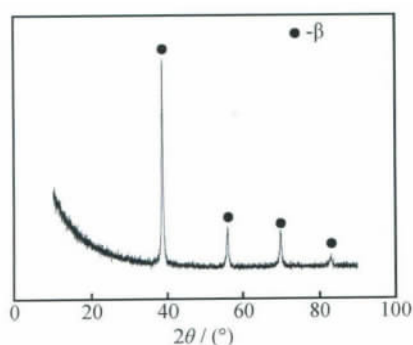
图 6 冷轧态合金在 650^\circ\text{C} 退火 90min 的 XRD 图谱
